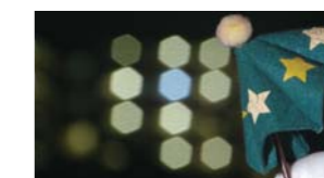
6-blade iris F5.6
